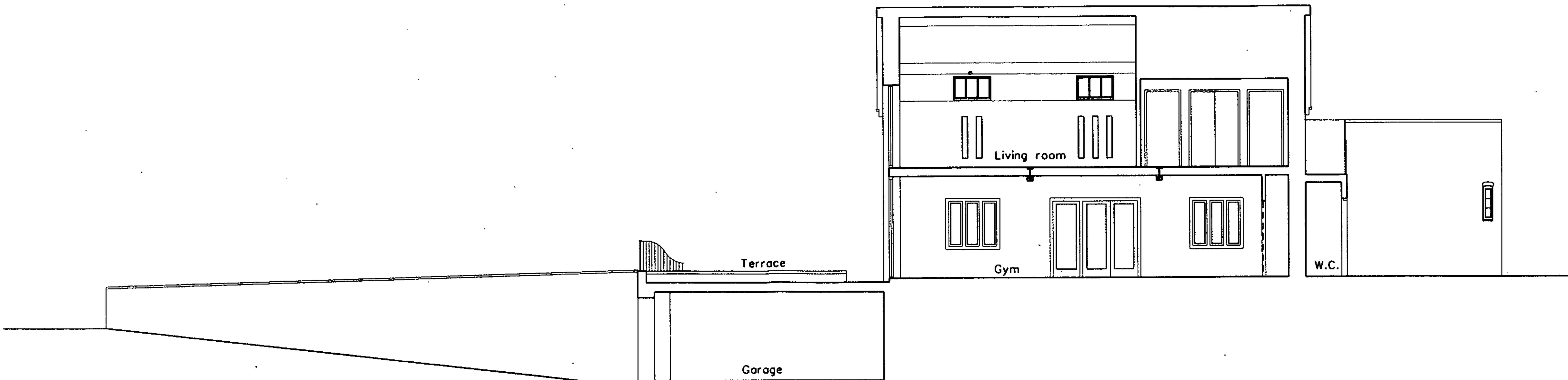
SECTION A-A
