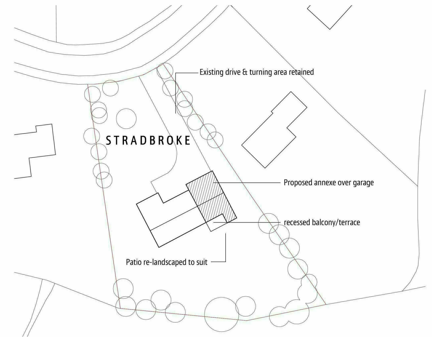
SITE PLAN 1:500
