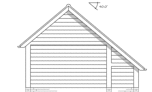
RIGHT ELEVATION
