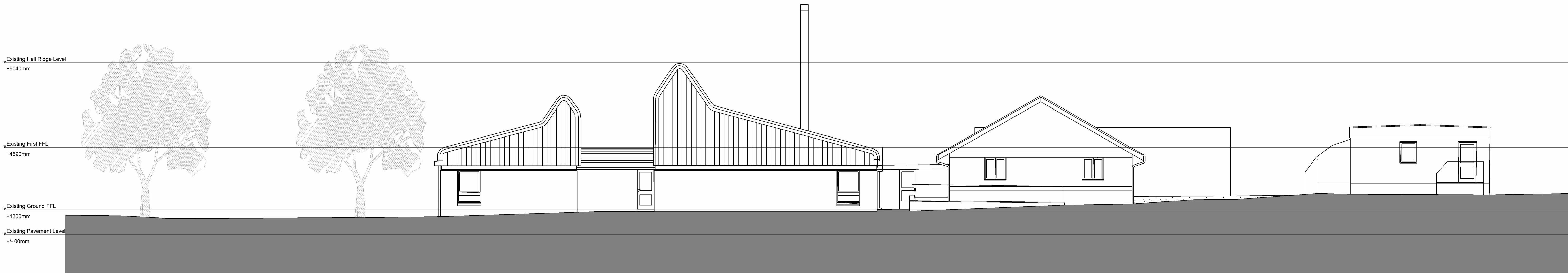
Elevation B 1:100
