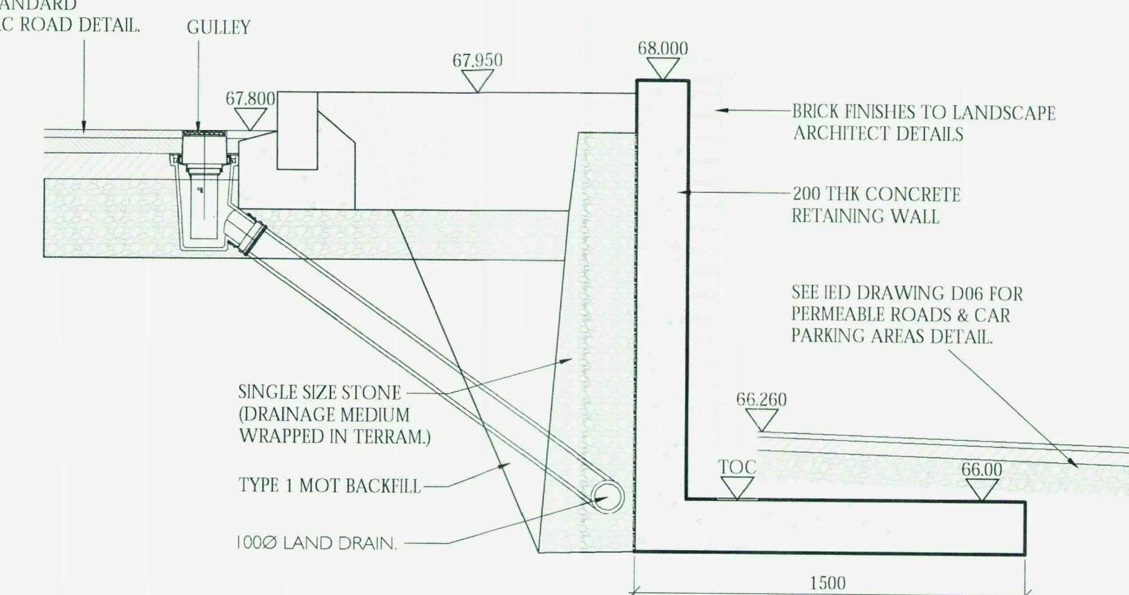
SECTION A-A 1:20
