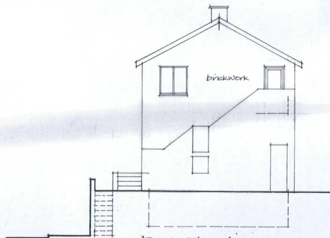
End Elevation (S.W.)
