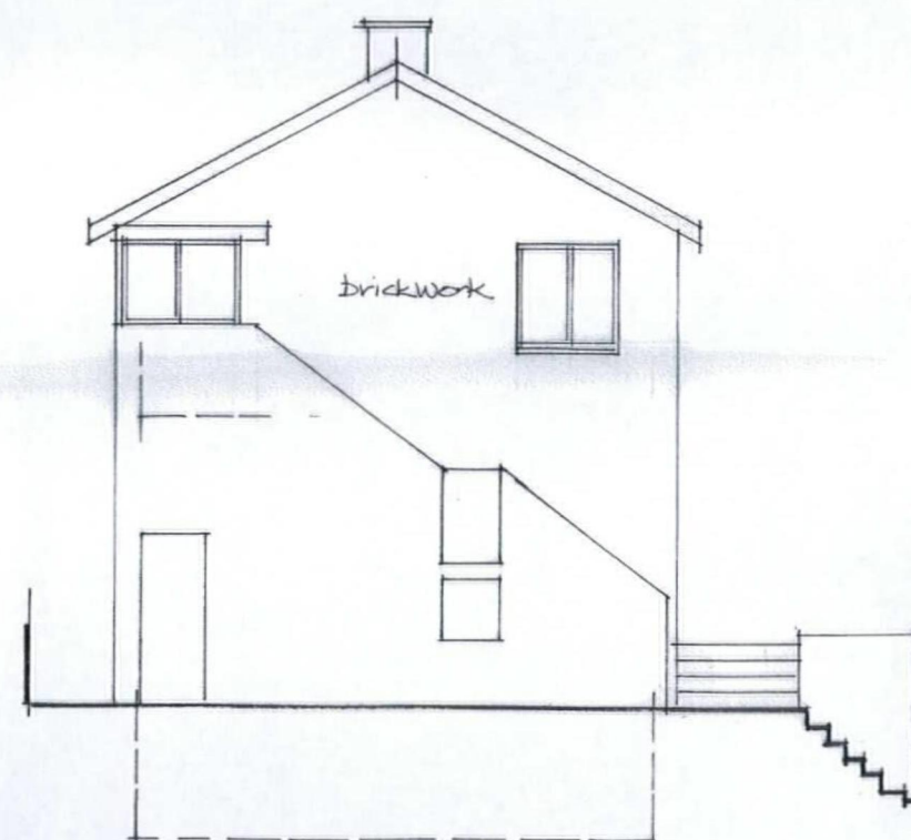
End Elevation (N.E.)
