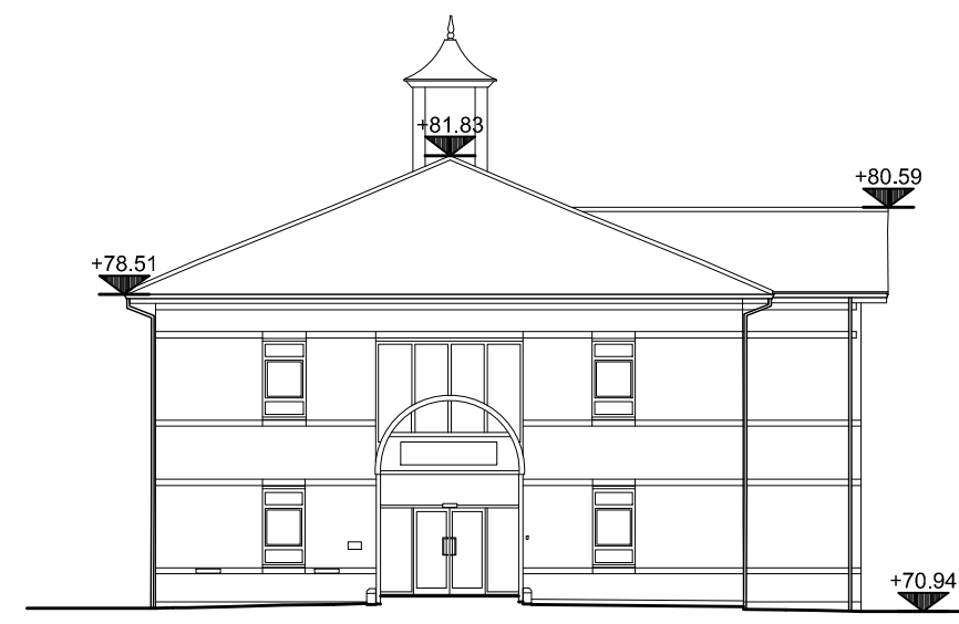
ELEVATION 4
