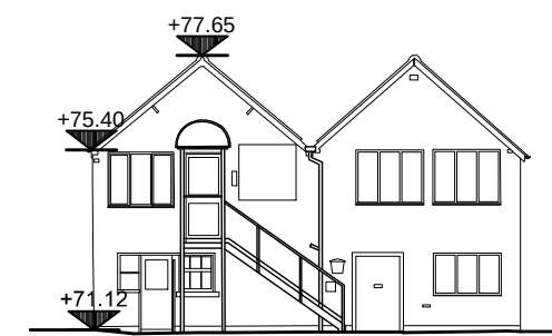
ELEVATION 07
