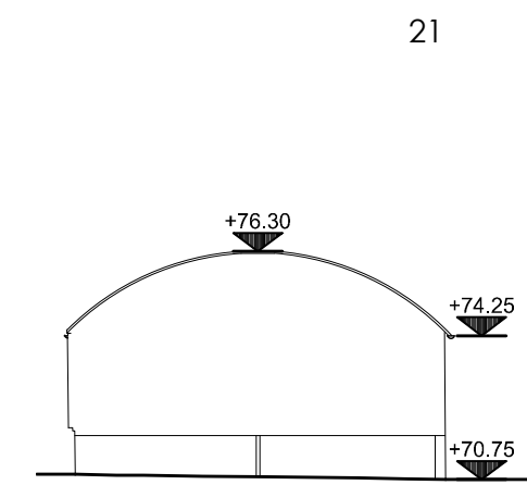
ELEVATION 12
