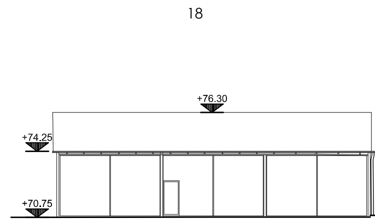
ELEVATION 13
