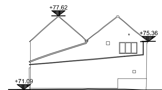
ELEVATION 09
