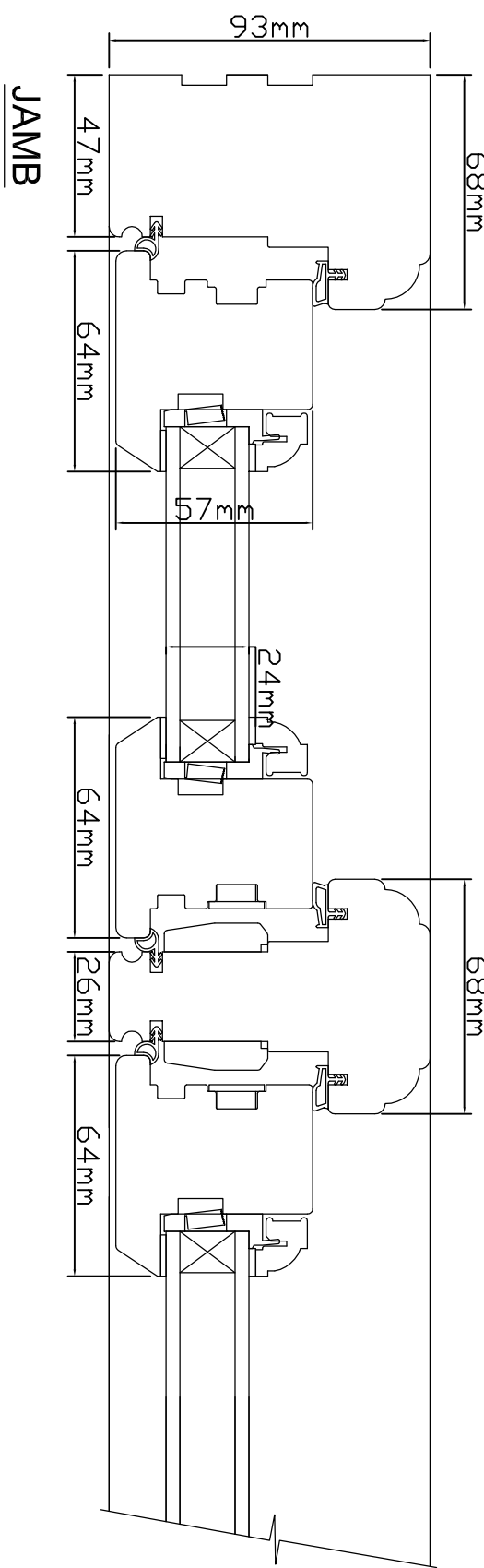
SECTION A-A
