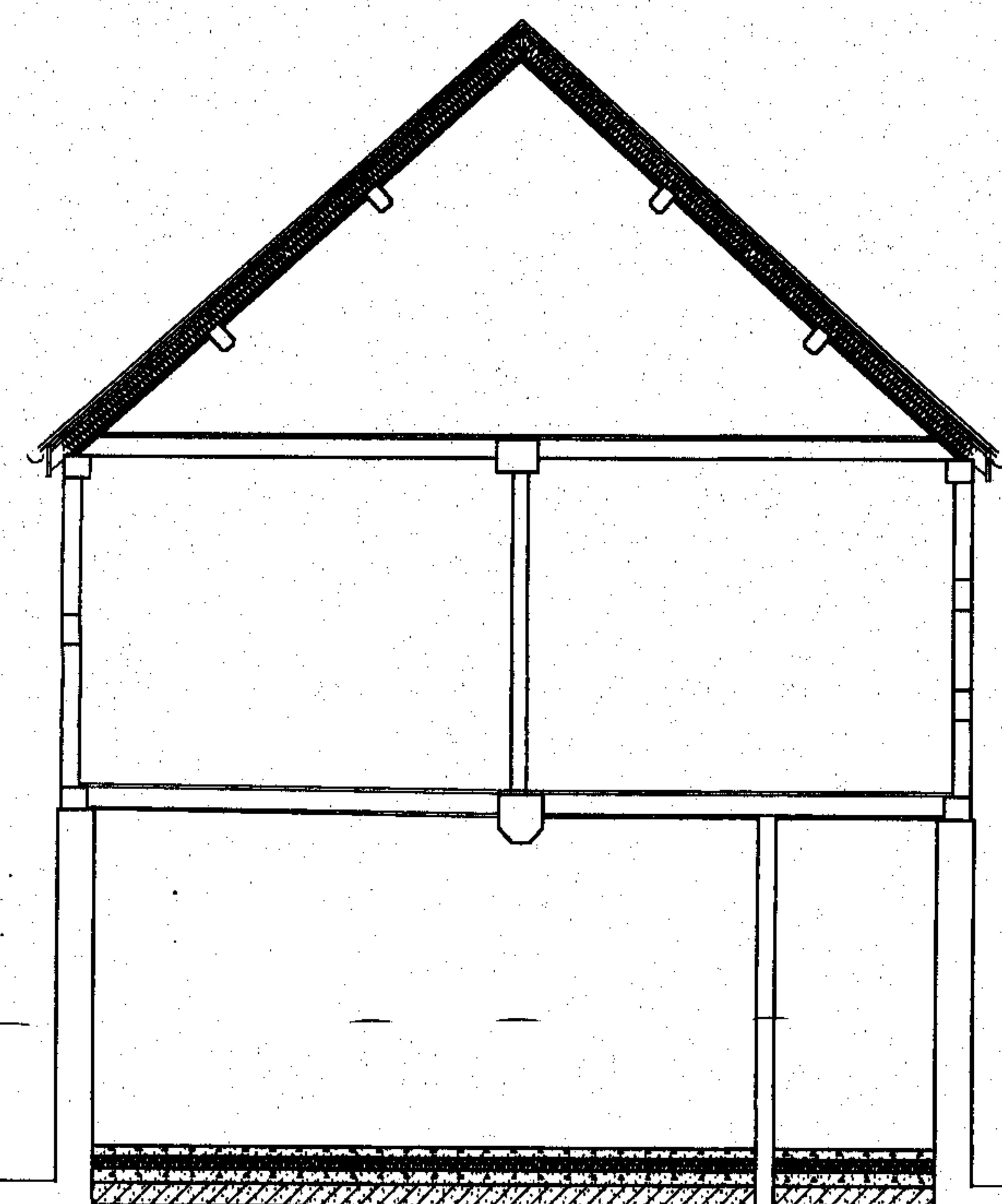
Section A-A
