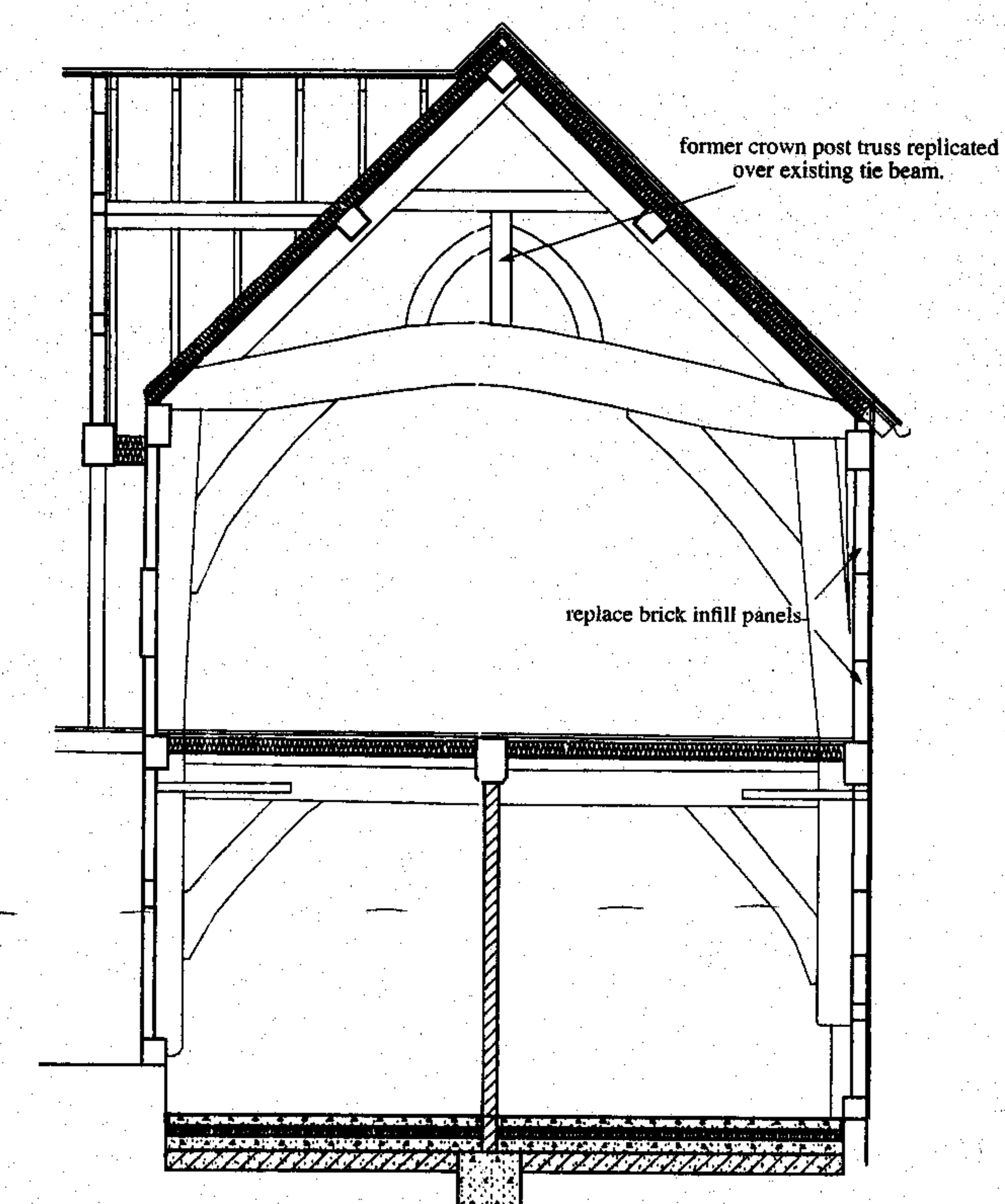
Section D-D
