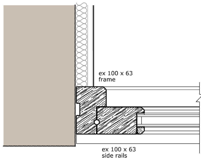
JAMB DETAIL - 1:5
