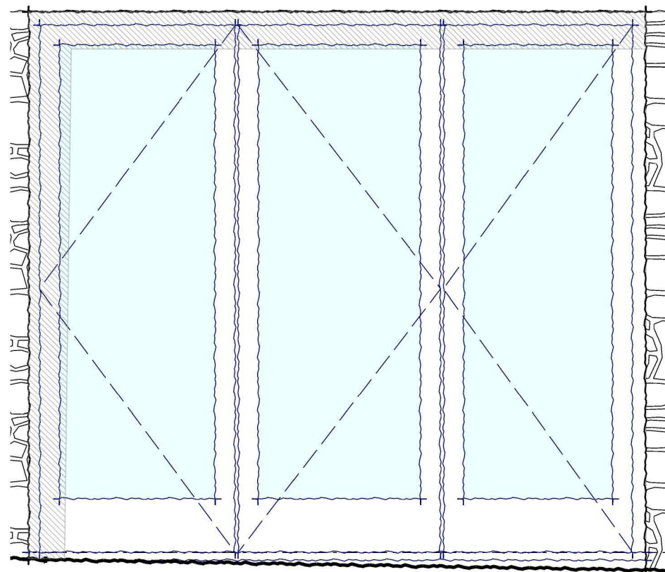
BI-FOLD DOOR ELEVATION - 1:10
