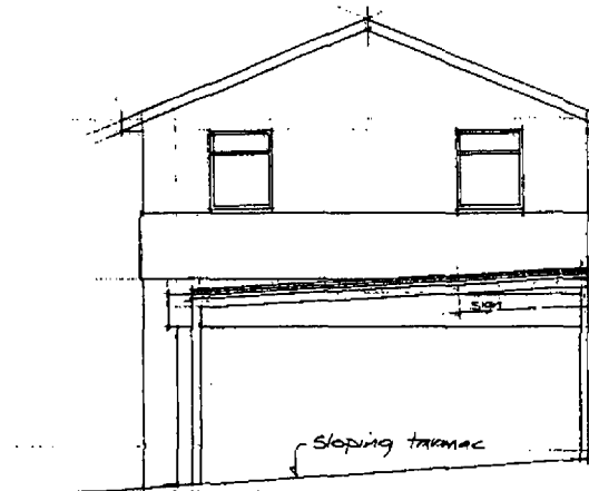
N.E. Elevation
